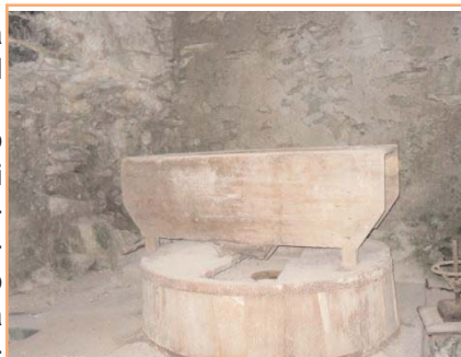
Macina, gru per sollevare le macine e ruota idraulica del Mulino Florio
